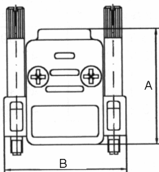
9-pol.
