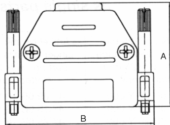
15/25/37/50 -pol.
