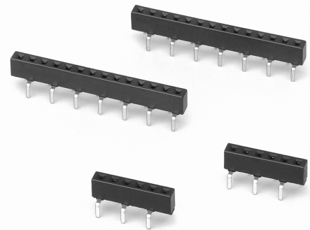
Doppelfederkontakt für Vierkantstift □ 0,635 mm Dual beam contact accepts square pin □ 0,635 mm
