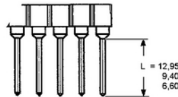
Serie 170/184 IC-Fassung und IC-Leisten mit Wire-Wrap-Kontakten IC-Socket and IC-Strips with Wire-Wrap-Contacts
