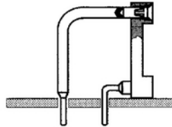
Serie 181 IC-Fassung für LED-Anzeigen IC-Socket for LED-Displays
